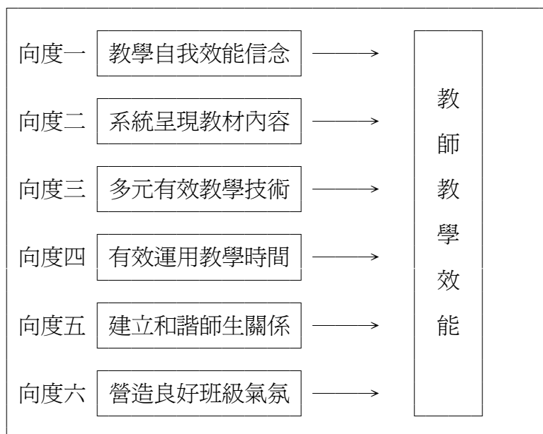
圖二 教師教學效能評鑑指標之建構圖
